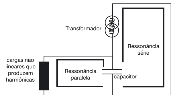
Diagrama Série-Paralelo
