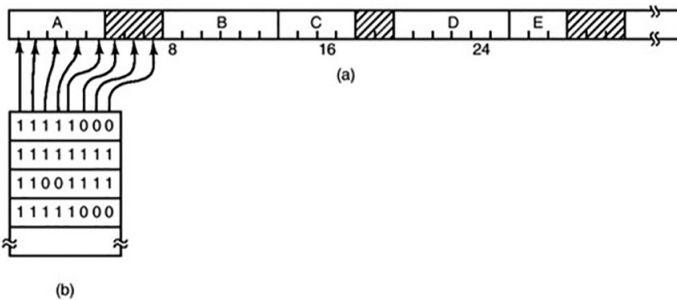
Figura 4.5 | Mapa de bits e uma parte da memória
