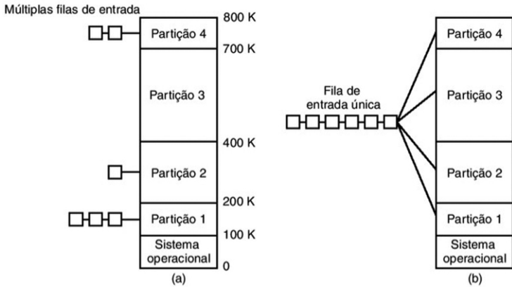
Figura 4.3 | Partições fixas com (a) múltiplas filas de entrada e (b) com uma única fila
