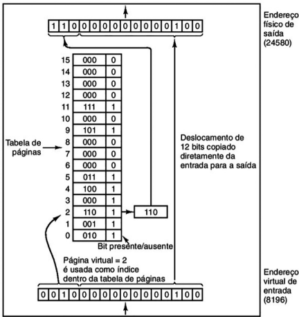
Figura 4.10 | Operação interna da MMU com 16 páginas
