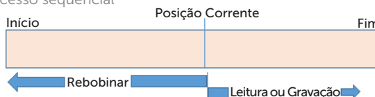
Figura 3.2 | Acesso sequencial
