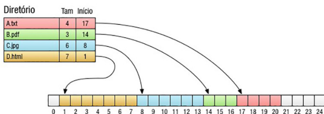
Figura 3.10 | Alocação Contígua
