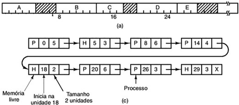
Figura 4.6 | Lista encadeada e uma parte da memória
