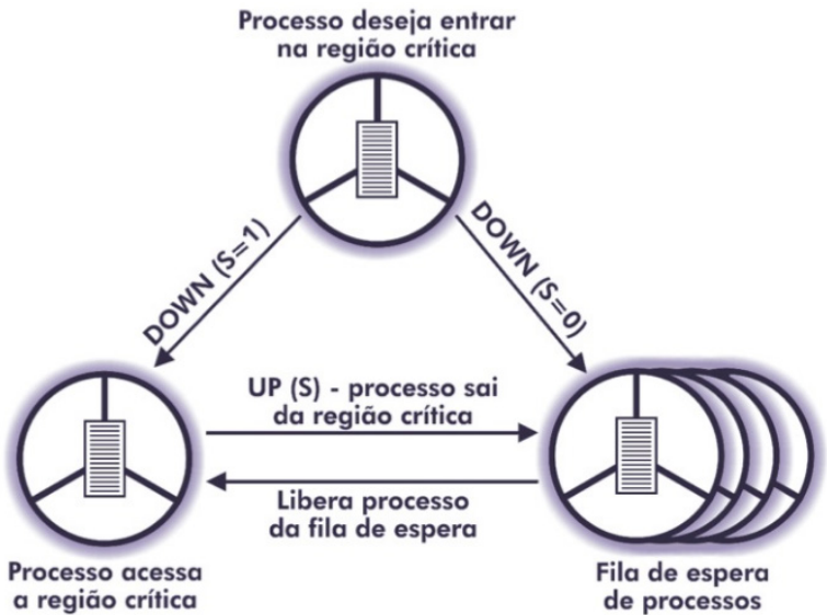
Figura 2.5 | Semáforo binário
