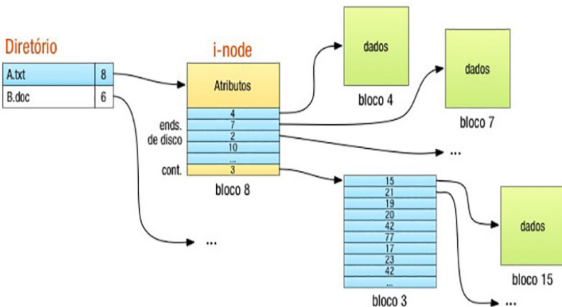
Figura 3.13 | I-nodes
