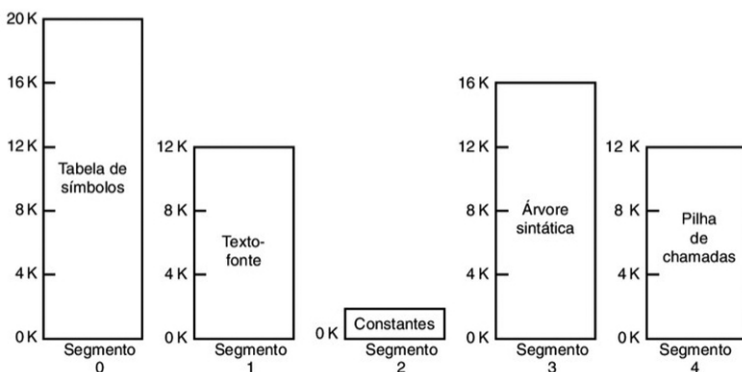
Figura 4.13 | Memória segmentada
