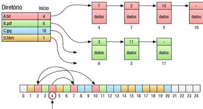
Figura 3.11 | Alocação por Lista Encadeada
