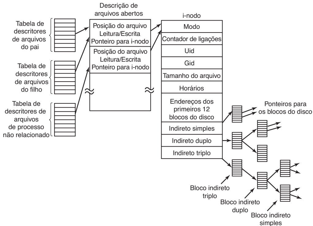
FIGURA 10.34 A relação entre a tabela de descritores de arquivos, a tabela de descritores de arquivos abertos e a tabela de i-nodos.
