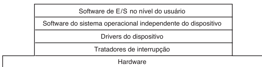
FIGURA 5.11 Camadas do sistema de software de E/S.
