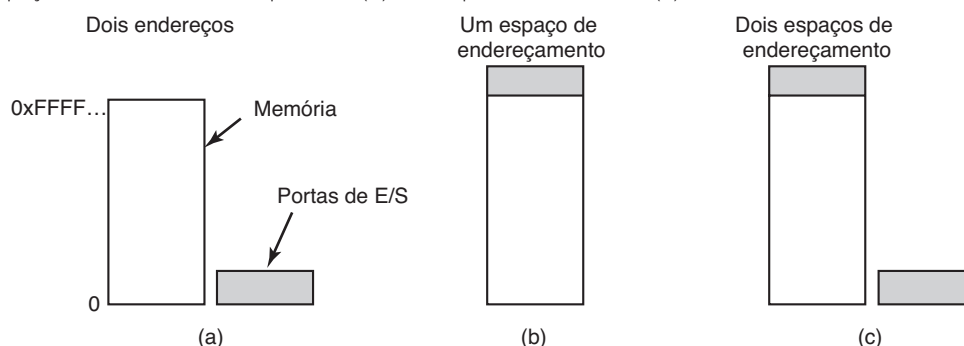
FIGURA 5.2 (a) Espaços de memória e E/S separados. (b) E/S mapeada na memória. (c) Híbrido.
